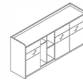
E902-2 W1621*D400*H805(mm)
