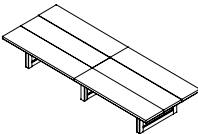
EF78 W4800*D1800*H760 W3600*D1600*H760
