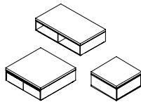
EF11 W1600*D900*H420 W1200*D1200*H420 W800*D800*H420
