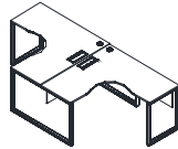
DL62-2.GJ W1400•D2812•H750 W1500•D3012•H750 W1600•D3212•H750
