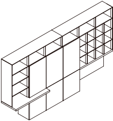
ED98 W3830*D560*H2130(mm)
