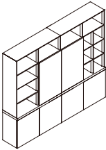
ED96 W2530*D430*H2130(mm)
