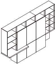
ED97 W3200*D560*H2130(mm)
