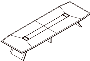
ED78 W4800*D1600*H760(mm)
