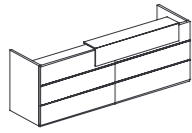
DL81(L/R)-2 W2886*D841*H1126
