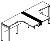
DE622FN-A 1400(W)*3020(D)*750(H) 1500(W)*3220(D)*750(H) 1600(W)*3420(D)*750(H)
