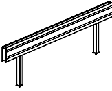
DEKHL 1200(W)*300(D)*40(H) 1300(W)*300(D)*40(H) 1400(W)*300(D)*40(H)
