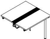
DE626FN 1400(W)*1420(D)*750(H) 1500(W)*1620(D)*750(H) 1600(W)*1620(D)*750(H)
