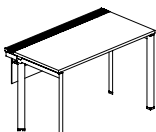
DE67FN 1400(W)*733(D)*750(H) 1500(W)*833(D)*750(H) 1600(W)*833(D)*750(H)
