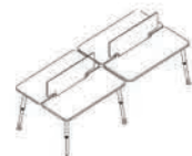
DW616 2800(W)*1210(D)*750(H) 3000(W)*1330(D)*750(H) 3200(W)*1410(D)*750(H)
