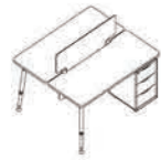
DW66 1400(W)*1210(D)*750(H) 1500(W)*1330(D)*750(H) 1600(W)*1410(D)*750(H)
