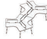
DW618 4720(W)*2710(D)*750(H)
