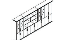
ER98 4046(W)*418(D)*2000(H)
